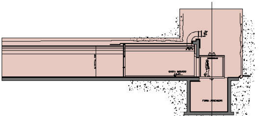
PARTICOLARE SEZIONE IMBARCO scala 1:200
