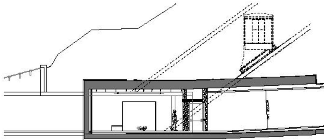
PARTICOLARE SEZIONE INGRESSO scala 1:200
