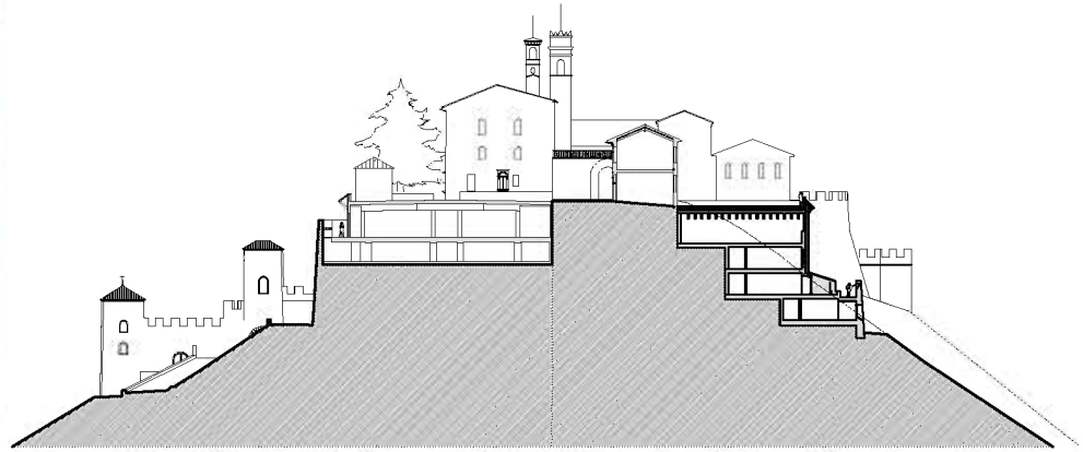
SEZIONE JUNIOR SUITES OVEST
