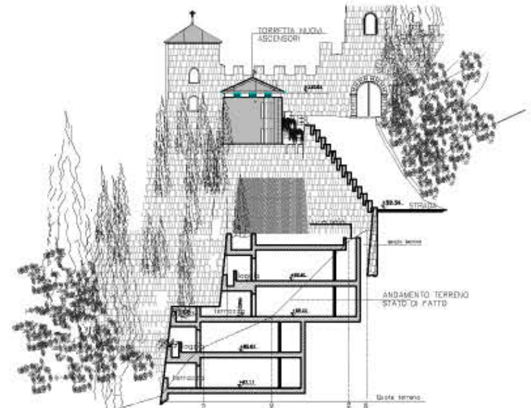
SEZIONE JUNIOR SUITES EST
