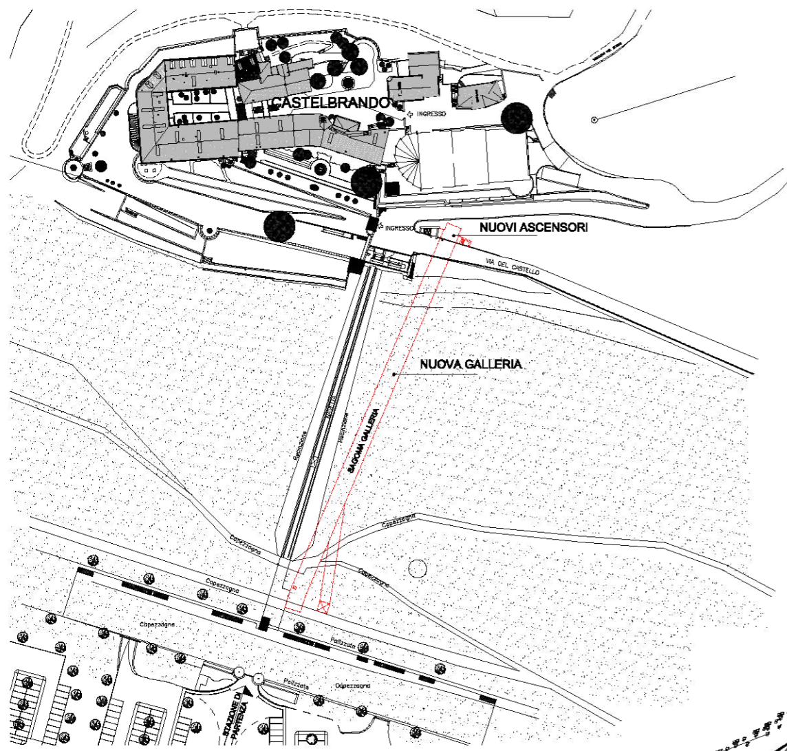
PLANIMETRIA GENERALE scala 1:2000
