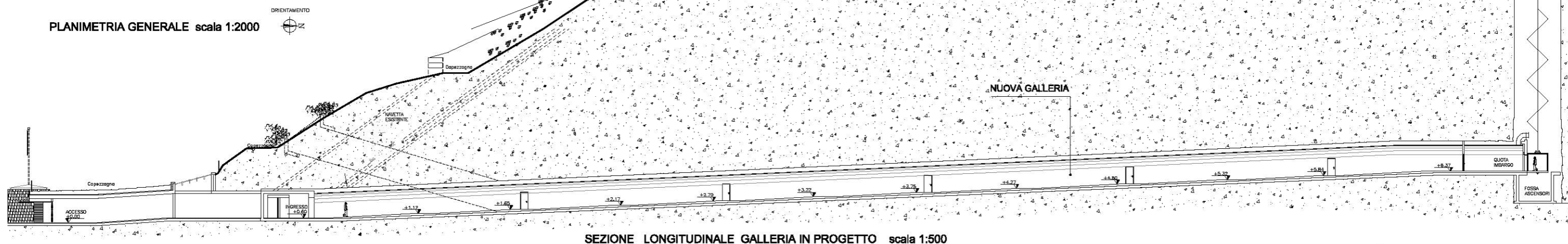
SEZIONE LONGITUDINALE GALLERIA IN PROGETTO scala 1:500
