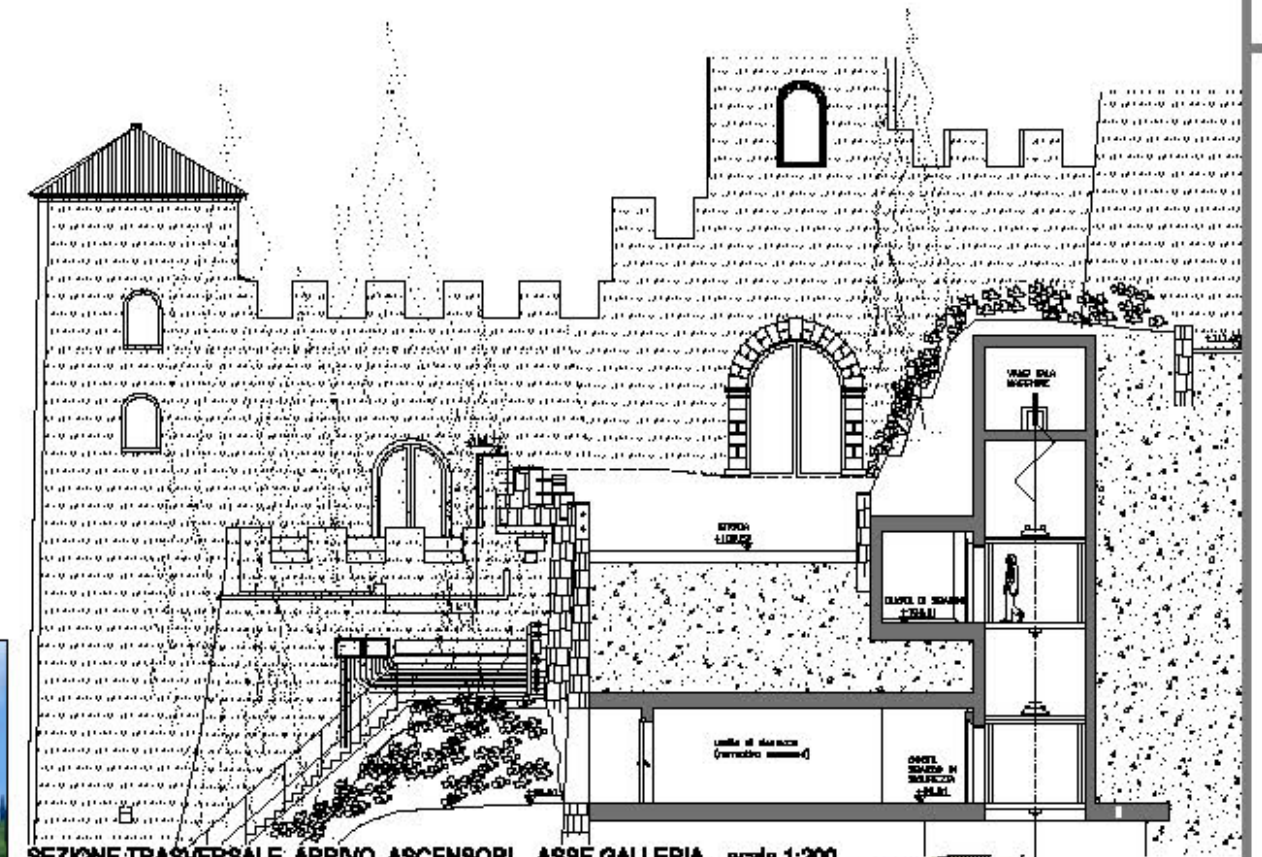
SEZIONE TRASVERSALE ARRIVO ASCENSORI ASSE GALLERIA scala 1:200
