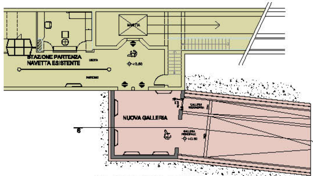
PARTICOLARE PIANTE INGRESSO scala 1:200
